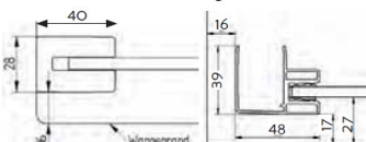
Einbausituation Wannenmontage:
