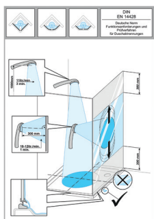
Duschabtrennung mit hohem Profil Hohe Dichtigkeit
