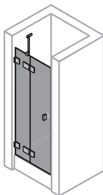
Schwingtür mit festem Segment
