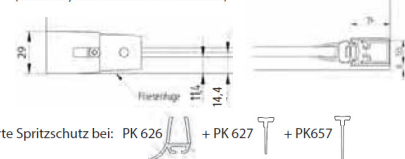
Einbausituation Bodenmontage: (Sondermaß, wenn außerhalb vom Produktmaß)
