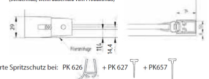
Einbausituation Bodenmontage: (Sondermaß, wenn außerhalb vom Produktmaß)
