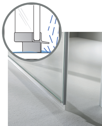
Duschabtrennung ohne Profil oder Schwallenschutzleiste Eingeschränkte Dichtigkeit
