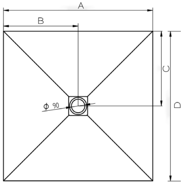
Ausführung rechteckig
